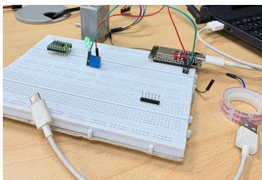
Montaje electrónico para prueba entre llantas y motores
